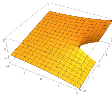
図 14: 虚部
