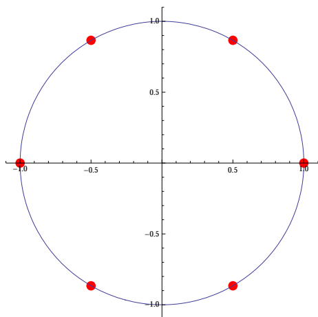
図 30: z^6 = 1 の解
