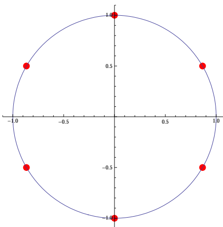
図 31: z^6 = -1 の解
